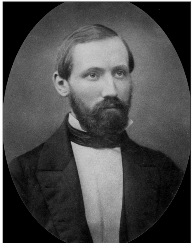
Bernhard Riemann (1826-1866)
